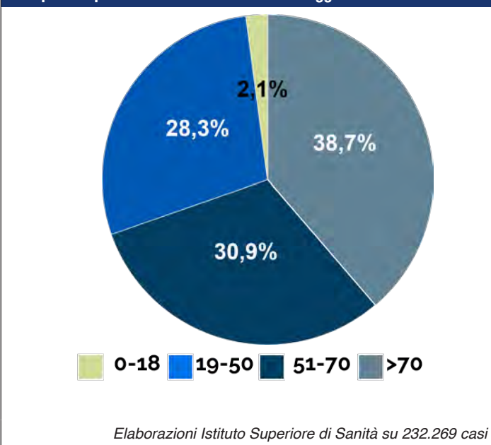
Casi positivi per fasce di età in Italia al 29 maggio 2020
